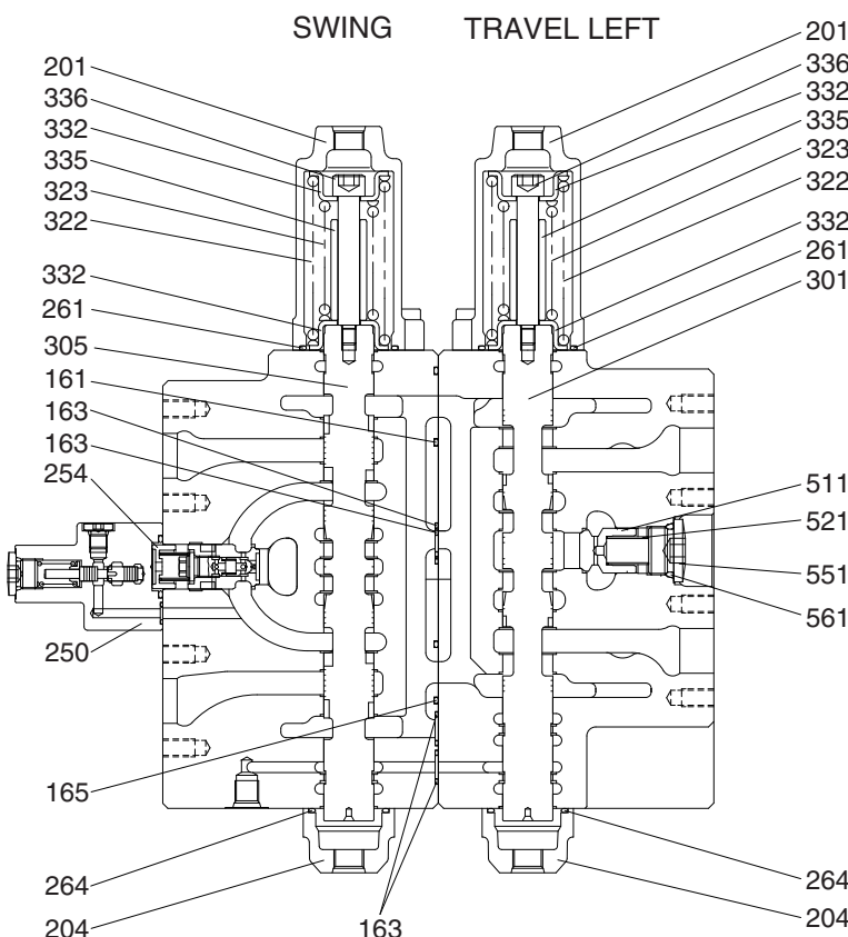
SECTION D-D
