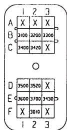
J1 CONEC. NEGRO DE 18 PINES (TODOS LOS ALAMBRES AZULES) J2 CONECTOR BLANCO DE 18 PINES (MAYORMENTE LOS ALAMBRES AZULES Y PÚRPURAS)
