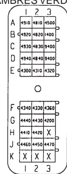
J4 CONECTOR BLANCO DE 30 PINES (MAYORMENTE LOS ALAMBRES VERDES)
