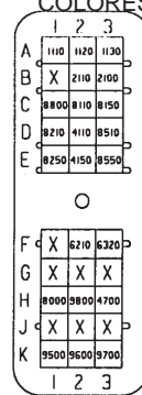
J3 CONECTOR NEGRO DE 30 PINES (ALAMBRES DE MÚLTIPLES COLORES)
