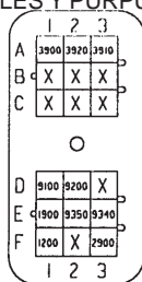
J1 CONEC. NEGRO DE 18 PINES (TODOS LOS ALAMBRES AZULES) J2 CONECTOR BLANCO DE 18 PINES (MAYORMENTE LOS ALAMBRES AZULES Y PÚRPURAS)
