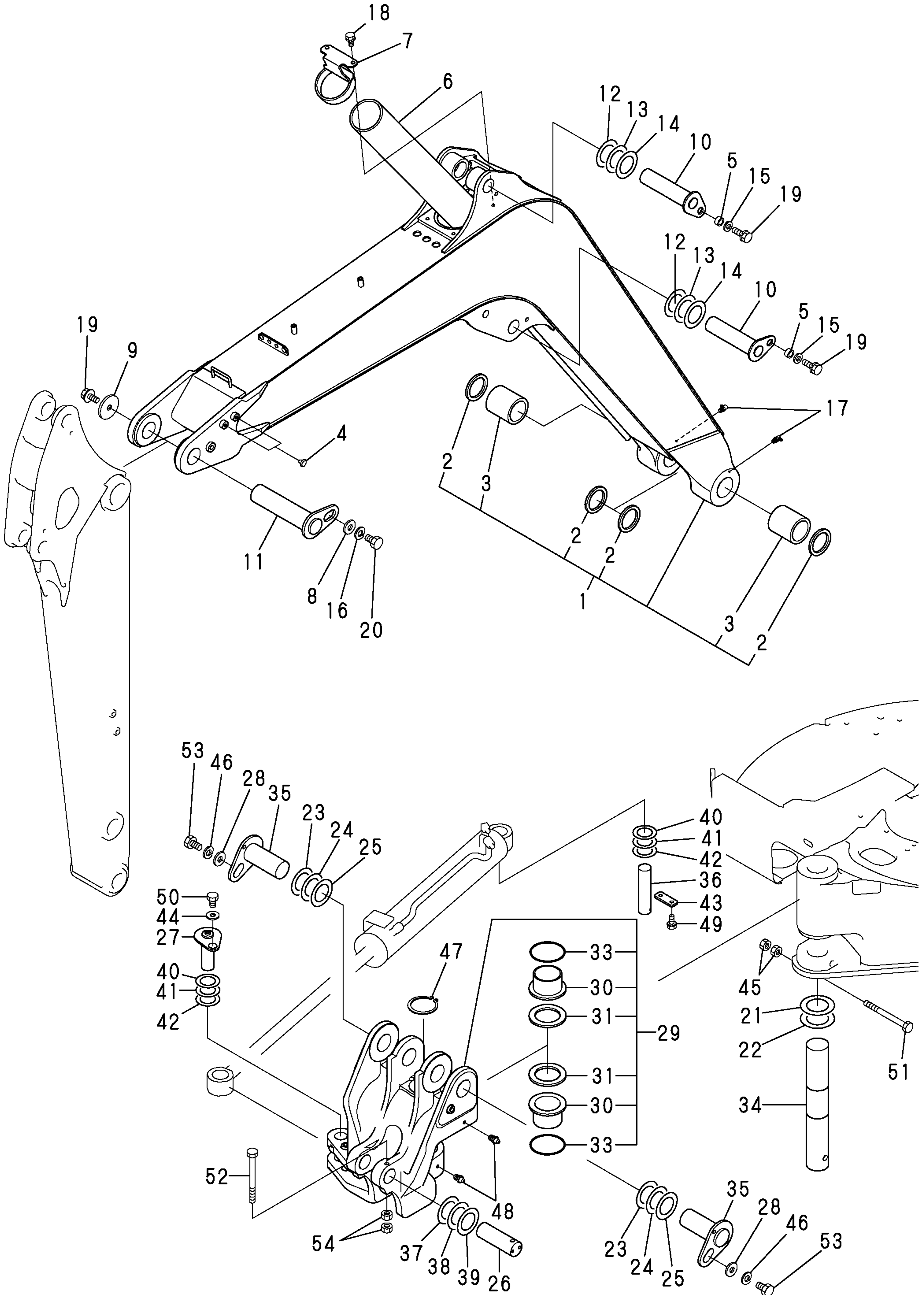
Fig. 53 BOOM & BOOM BRACKET
