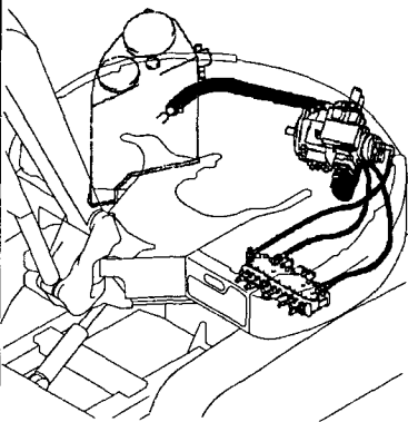
Fig.67 油圧配管 (バルブ~モータ、ブーム) HYD.OIL PIPING (VALVE ~ MOTOR, BOOM)
