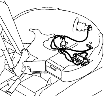
Fig.72 油圧配管 (PTOバルブ、 フレーム) (旧形) HYD.OIL PIPING (P.T.O. VALVE, FRAME) (PREVIOUS)
