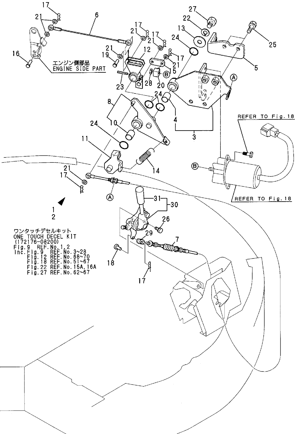
Fig. 9 アクセル (ワンタッチデセル) ACCELERATOR (ONE TOUCH DECEL)
