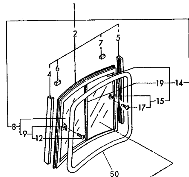
Fig. 40 キャビン (2) (サッシ) CABIN (2) (SASH)
