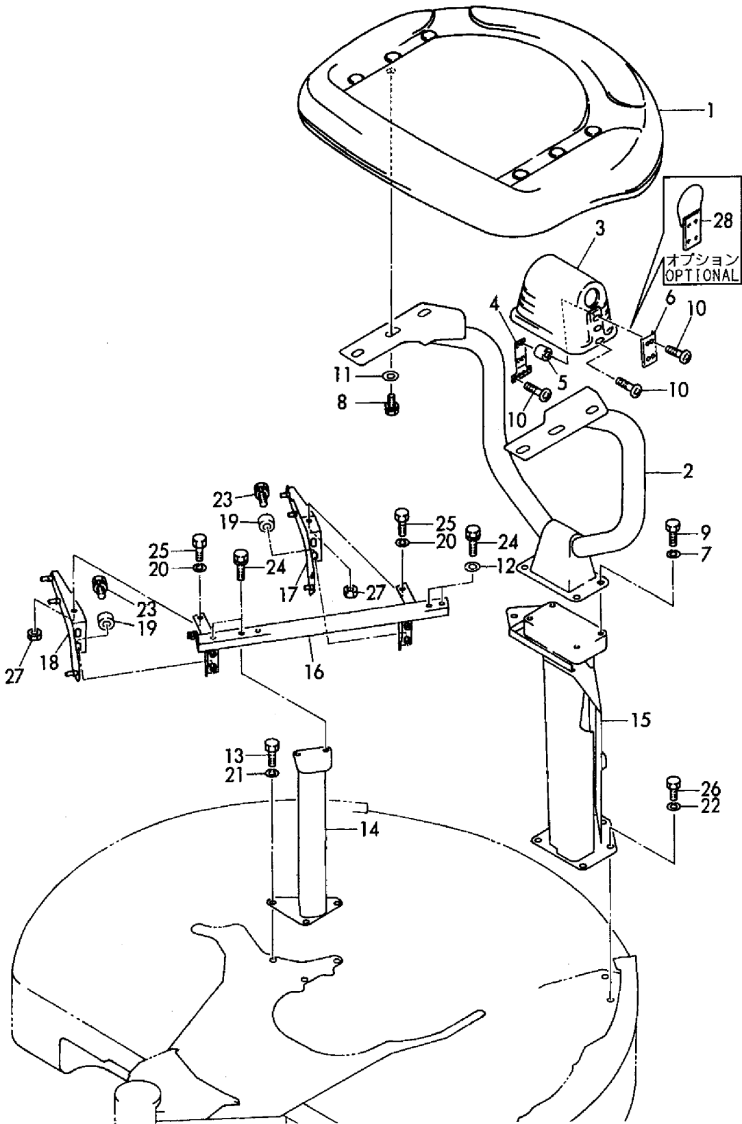
Fig. 43 キャノピ&キャノピフレーム CANOPY & CANOPY FRAME
