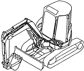
Fig. 50 HYD.OIL PIPING (P. T. O.)
