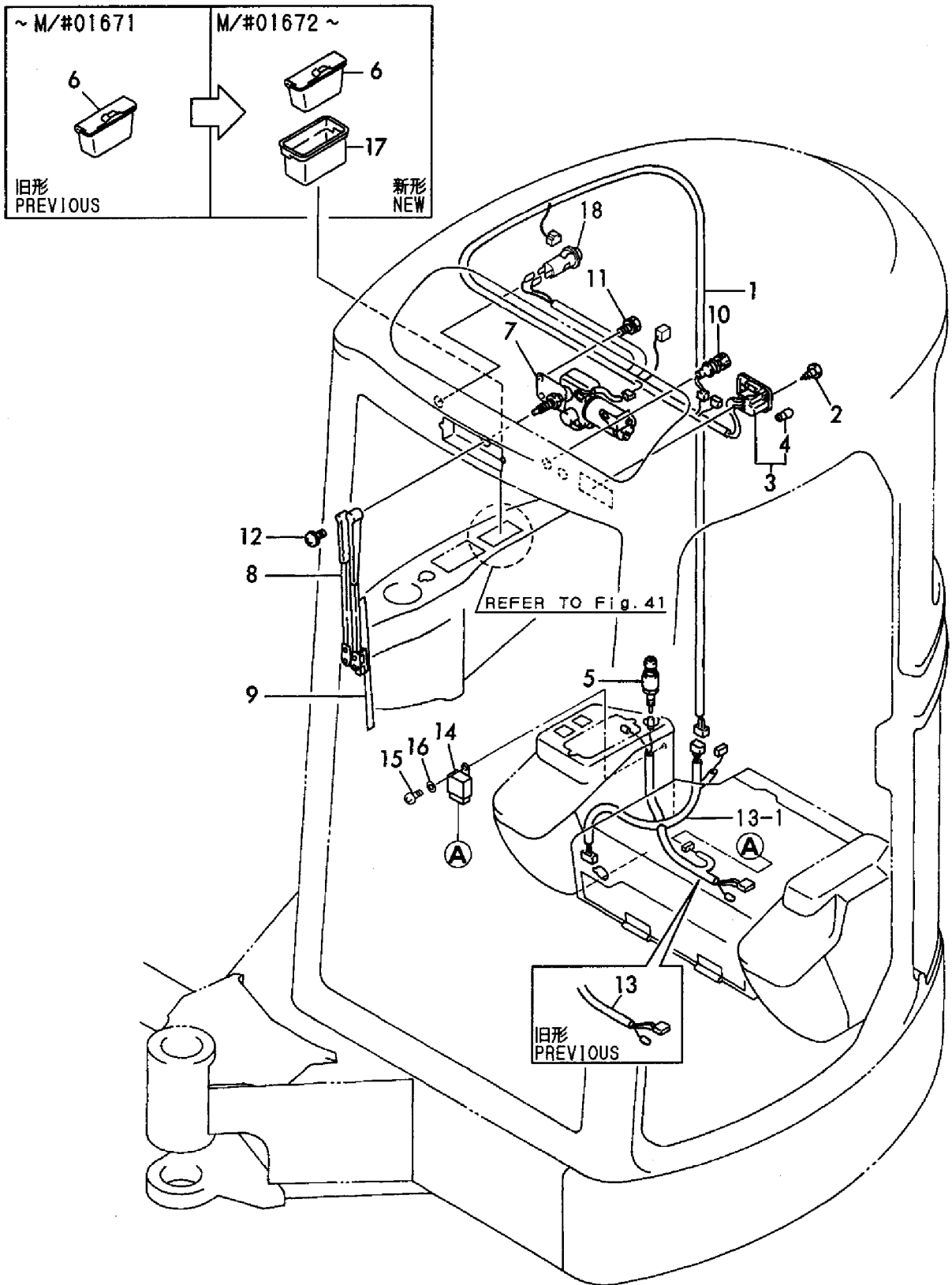
Fig. 19 電装品 (キャビン) ELECTRIC PART (CABIN)
