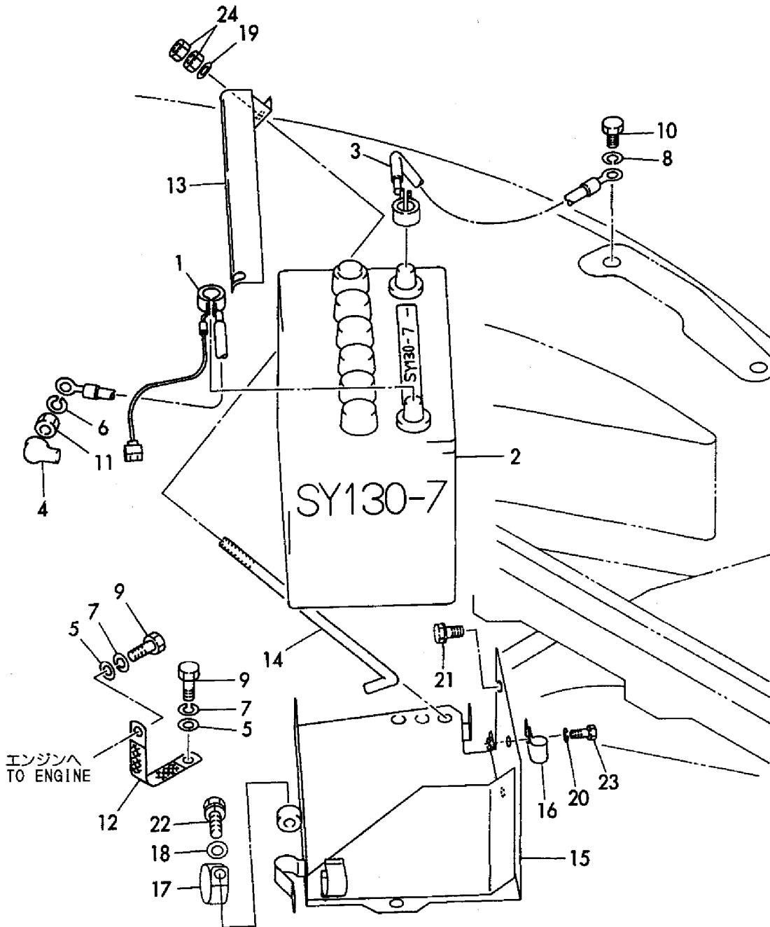
Fig. 16 バッテリ BATTERY
