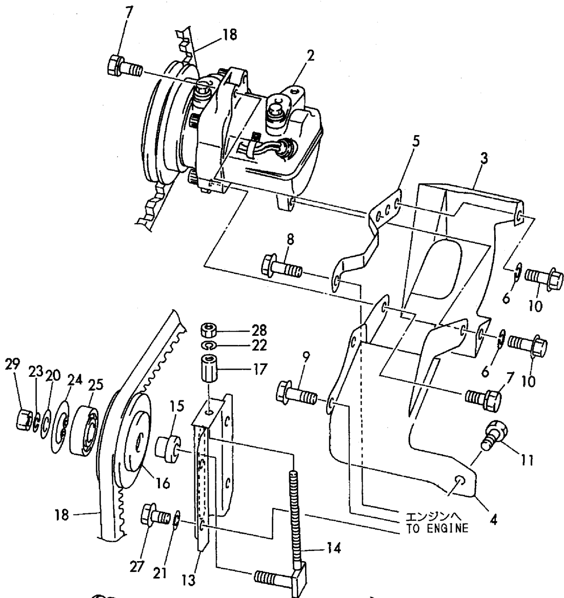
Fig. 11 コンプレッサー&Vプーリ (クーラ仕様) COMPRESSOR & V PULLEY (COOLER SPEC.)
