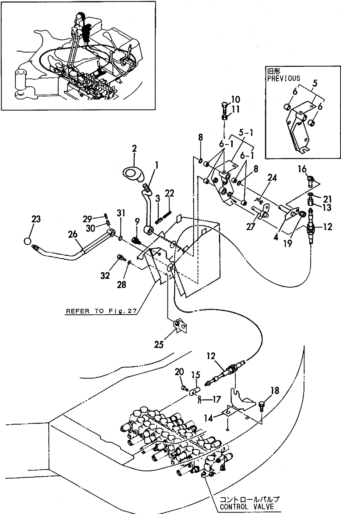
Fig. 30 操縦装置 (ブレード) CONTROL EQUIP. (BLADE)
