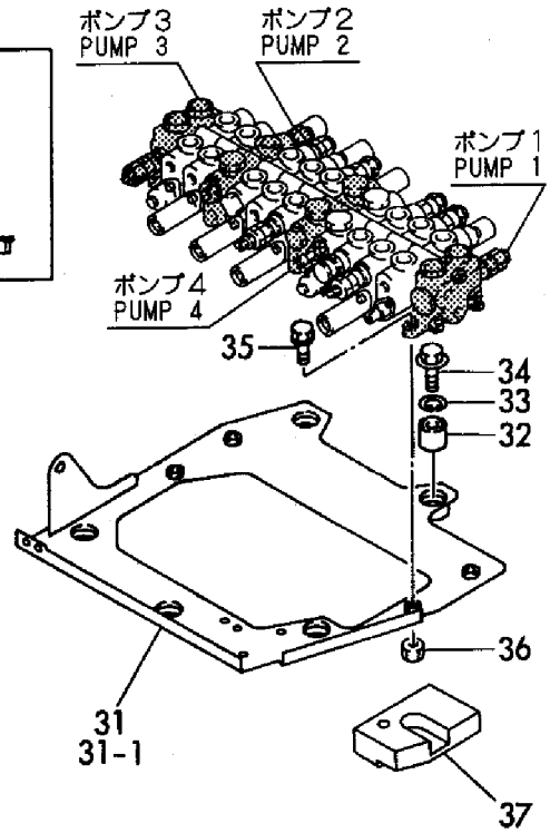
Fig. 60 コントロールバルブ (Pポート) CONTROL VALVE (P PORT)
