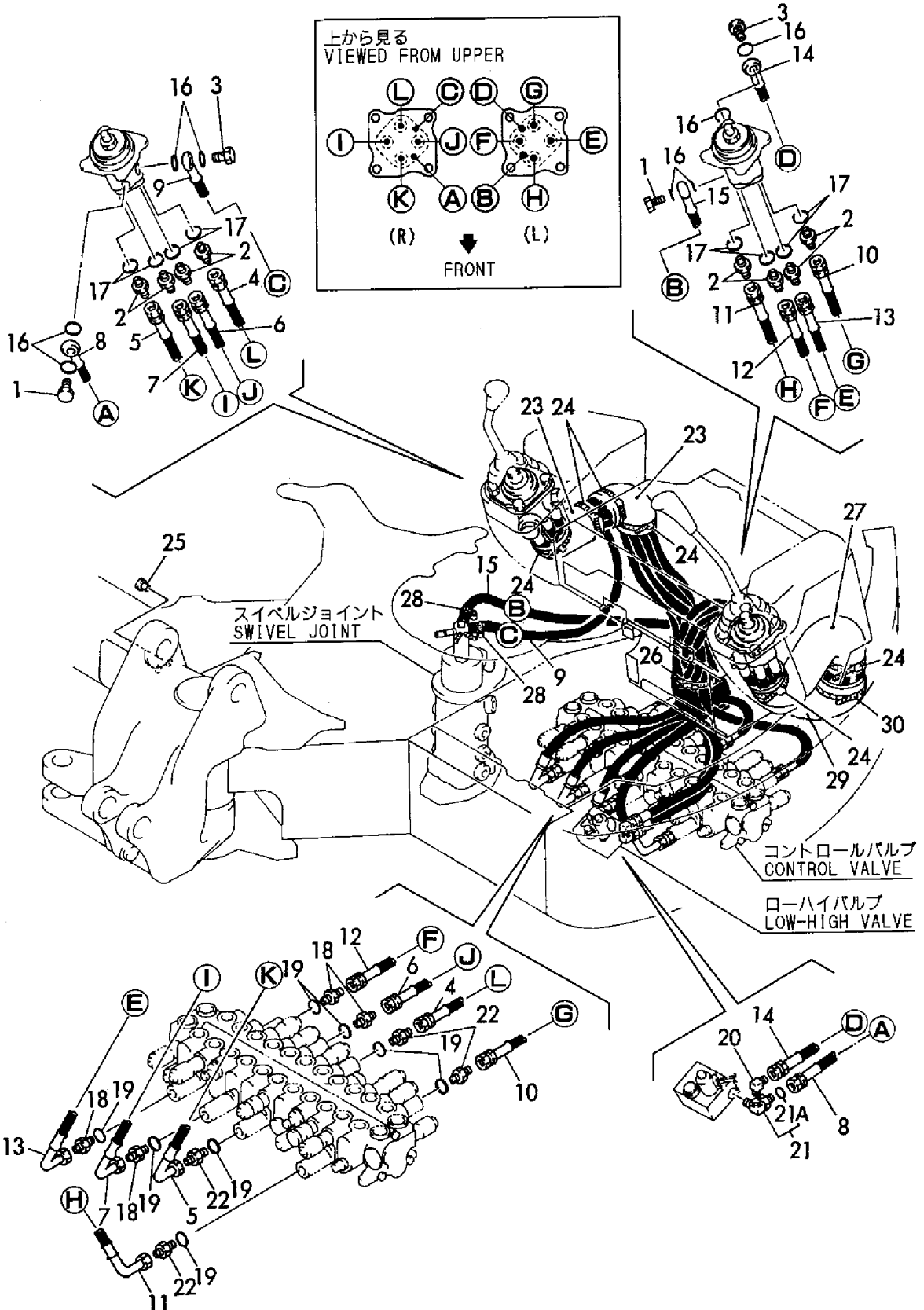
Fig. 88 コントロール配管 (ダイレクト) (旧形) CONTROL PIPING (DIRECT) (PREVIOUS) ~M/#01186
