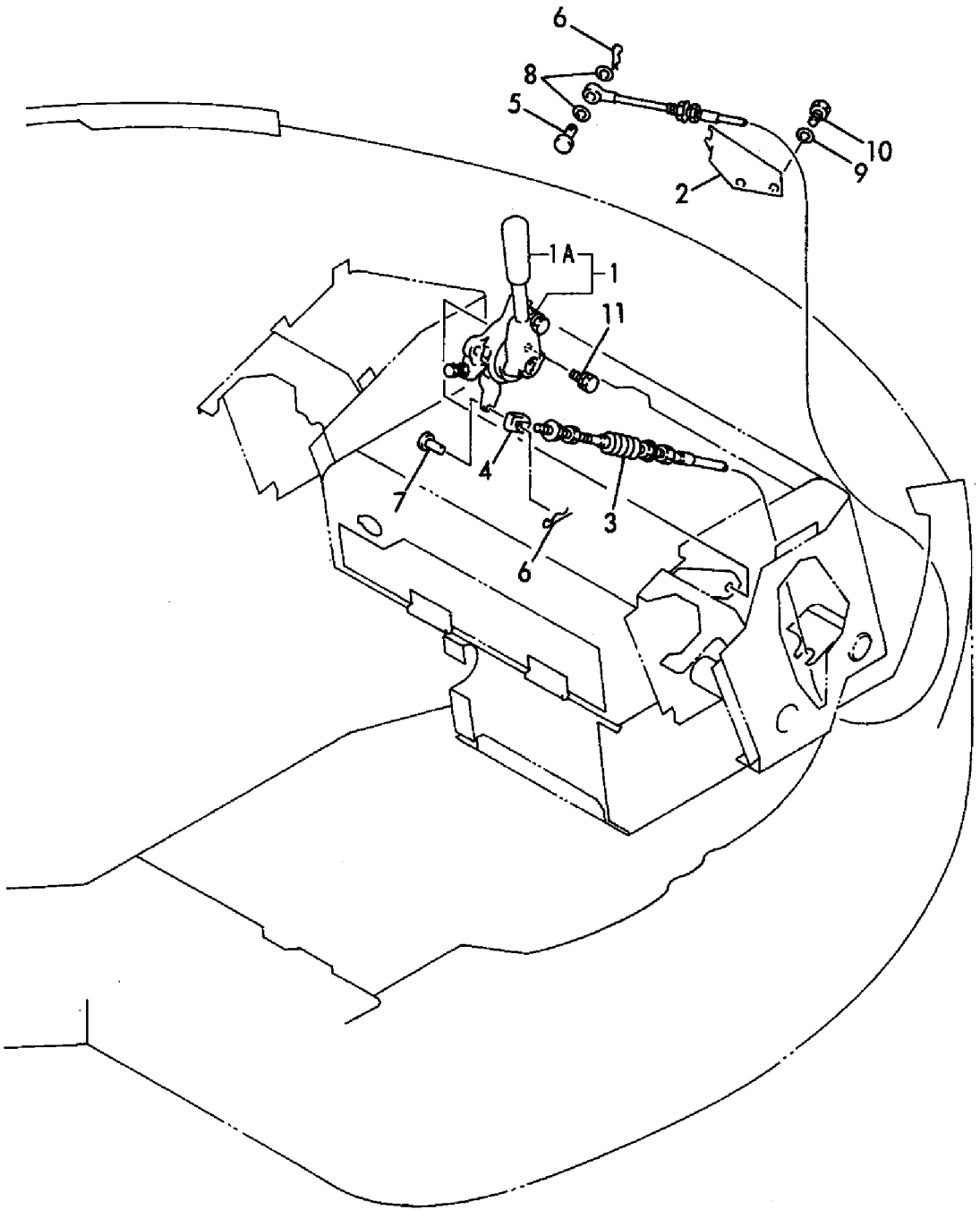
Fig. 8 アクセル ACCELERATOR
