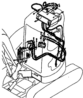
Fig.14 カバー (クーラー仕様) COVER (COOLER SPEC.)
