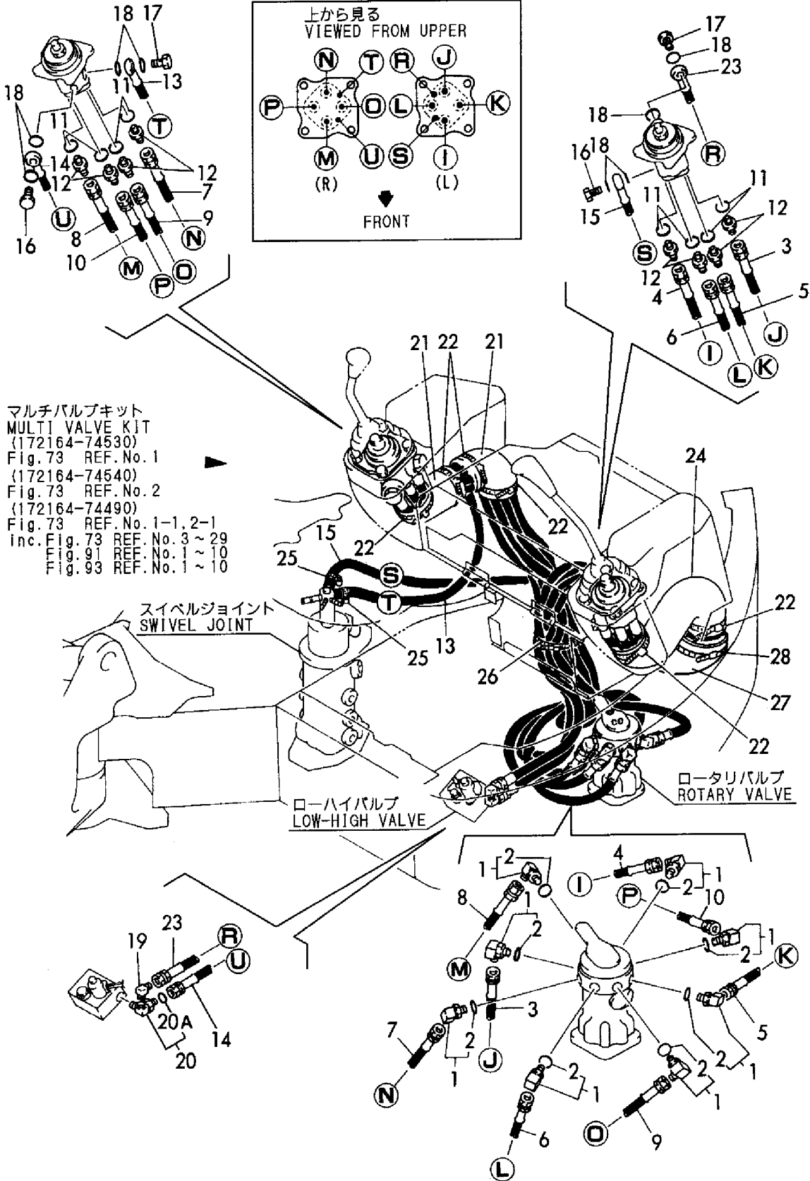
Fig. 91 コントロール配管 (リモコンバルブ~ロータリバルブ) (旧形) CONTROL PIPING (REMO.-CON. VALVE ~ROTARY VALVE) (PREVIOUS)
