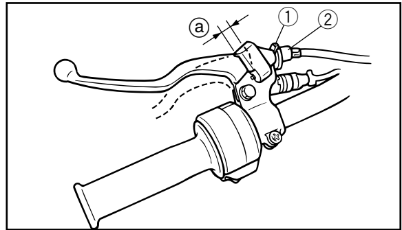
a. Free play 1. Locknut
