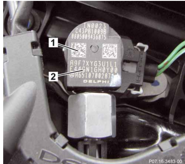
Piezo injector
