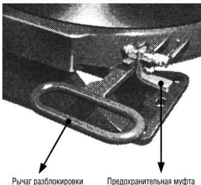
Рычаг разблокировки
