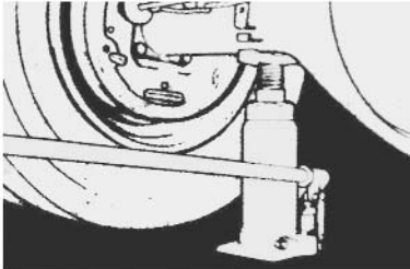
Установка домкрата под задний мост
