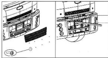
Установка домкрата под задний мост
