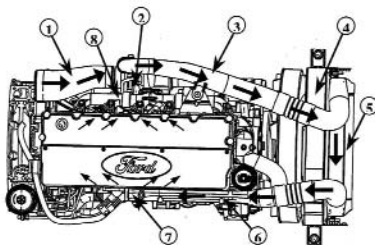
Схема работы промежуточного теплообменника (вид сверху)
