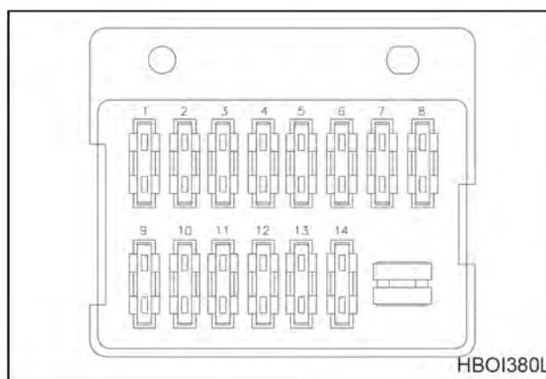
Рис. 104. БЛОК ПРЕДОХРАНИТЕЛЕЙ 1
