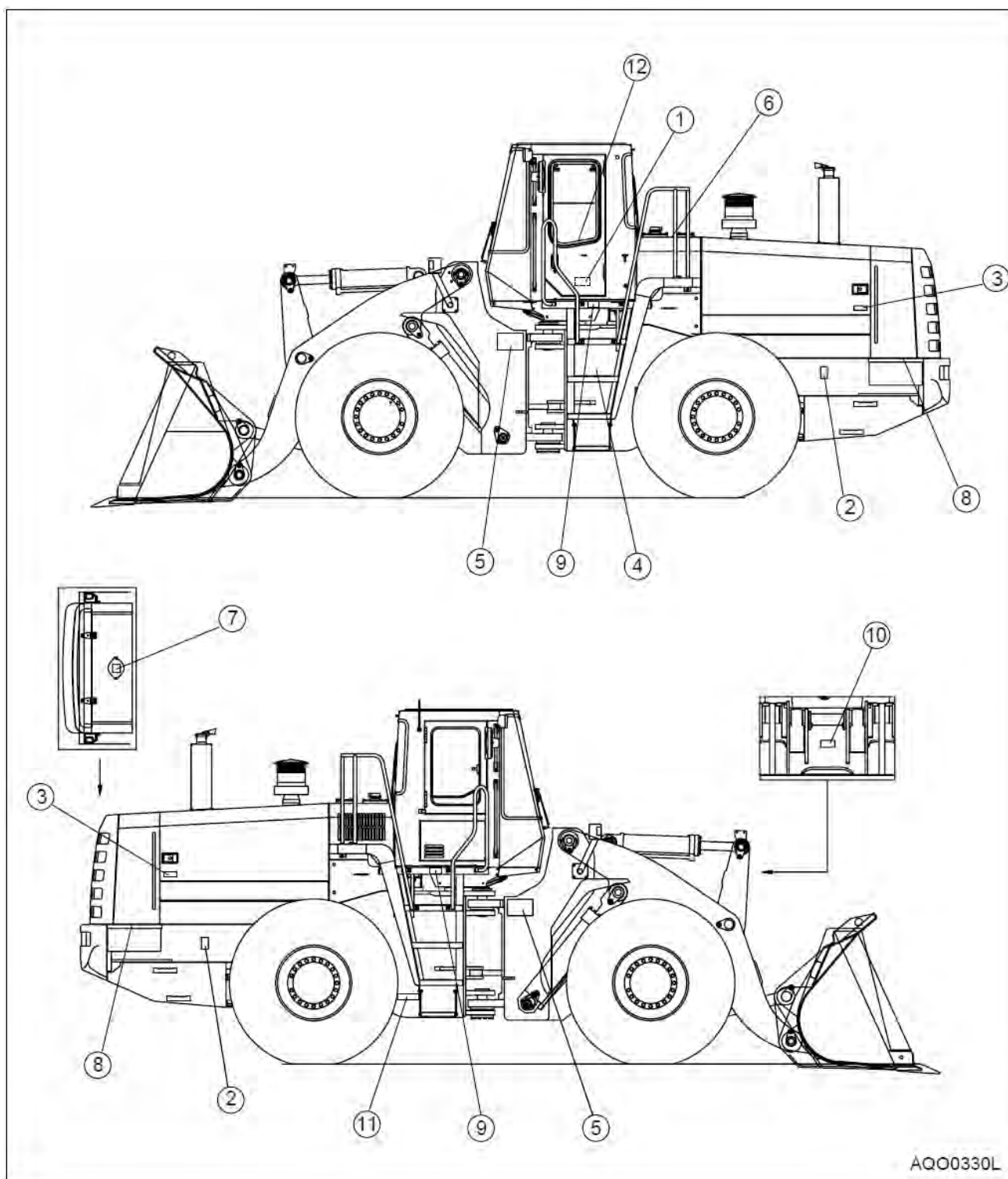
Рис. 2. Машина с кабиной
