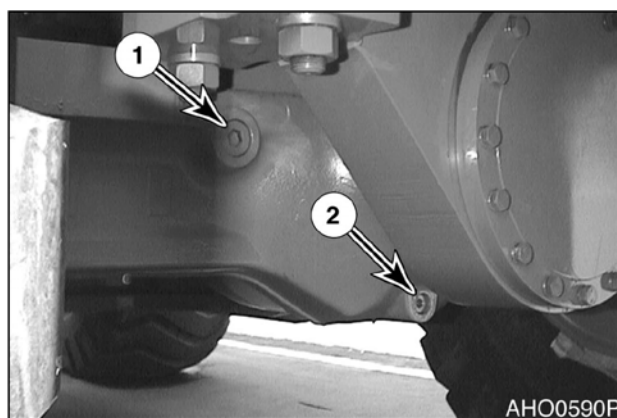
Рис. 78. ЗАДНИЙ МОСТ
