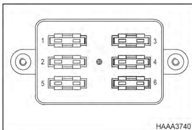
Рис. 105. БЛОК ПРЕДОХРАНИТЕЛЕЙ 2
