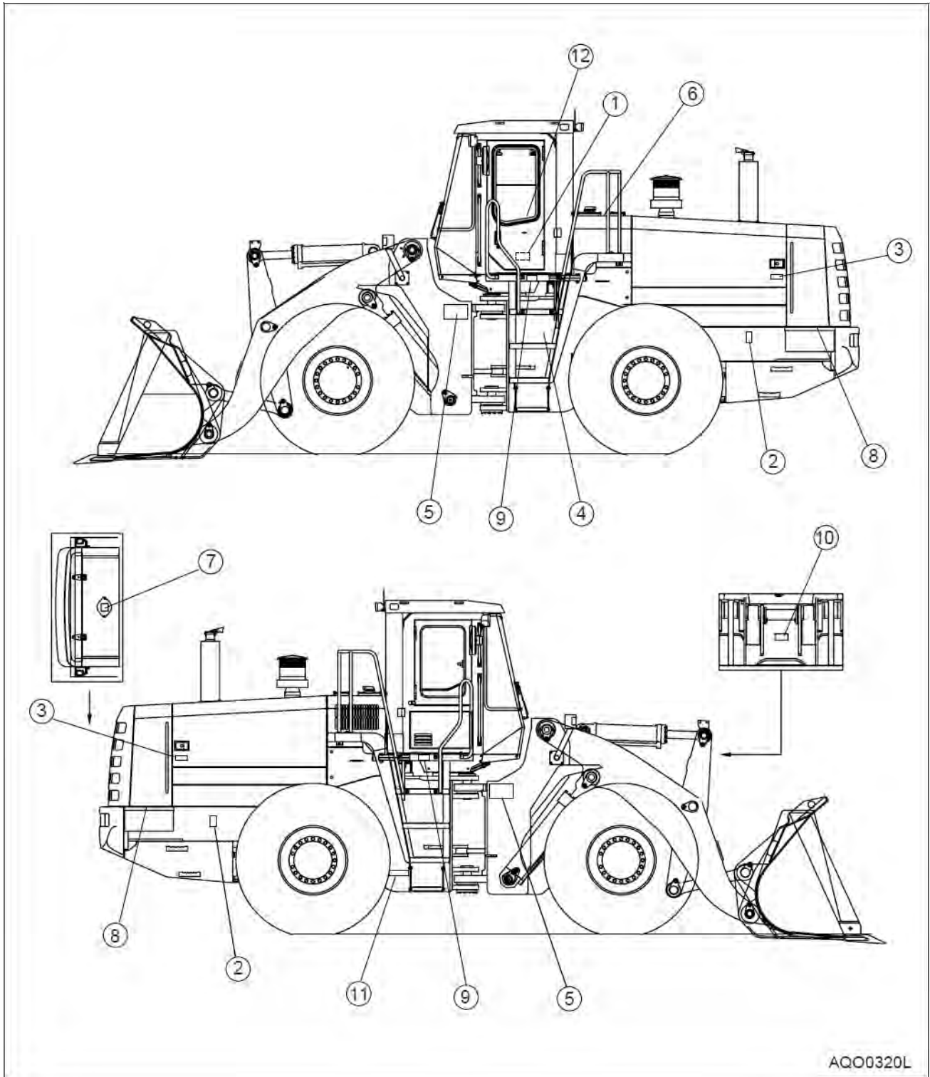
Рис.1. Машина с ограждением ROPS и кабиной
