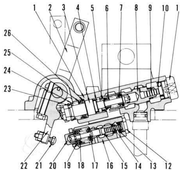
Разрез А-А
