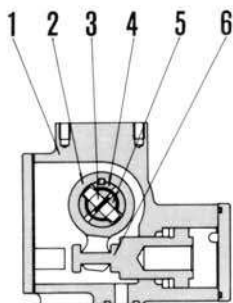
Разрез В-В
