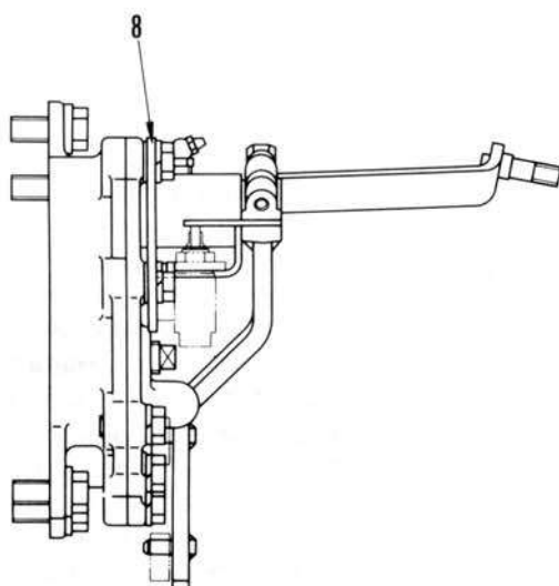
Вид Z
