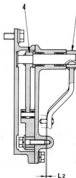
Сечение A-A
