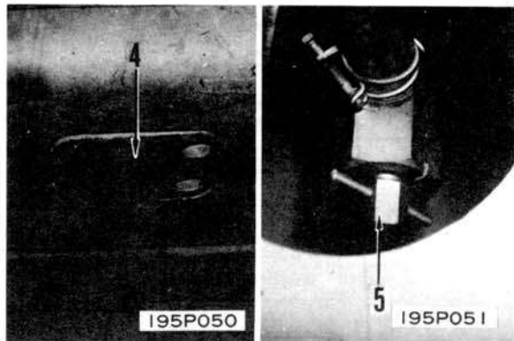
Стандартная машина
